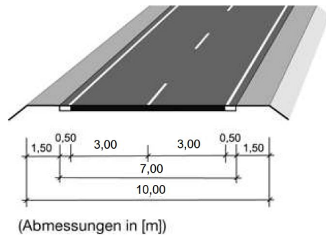
Regelquerschnitt nach „Richtlinien für die Anlage von Landstraßen“ (RAL)
